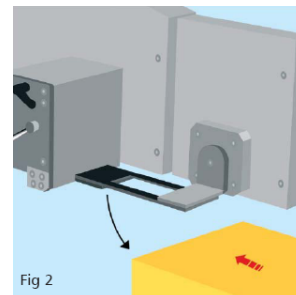
Fig 2 Applicateur type F : haute cadence, temps réel, sur la face avant ou arrière de produits en mouvement
