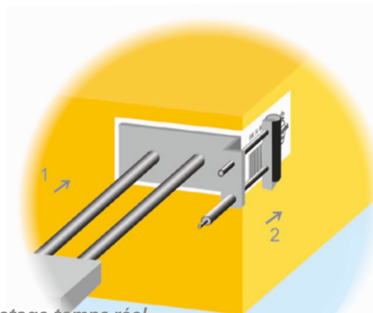
Type TE : Etiquetage temps réel Applicateur télescopique avec dispositif d'application en angle
