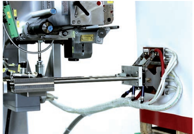
La tête d'application du QTB aspire l'étiquette découpée et active la colle
